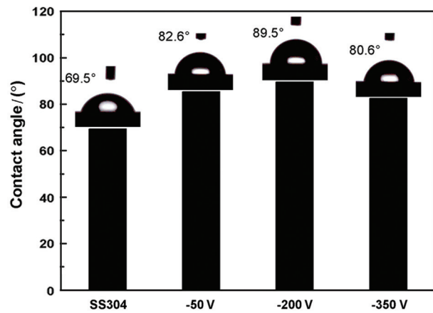
图9 基体和非晶碳膜与去离子水间的接触角
