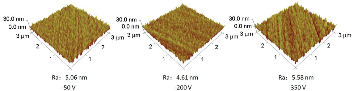
图 3 不同偏压非晶碳膜 AFM 形貌图
