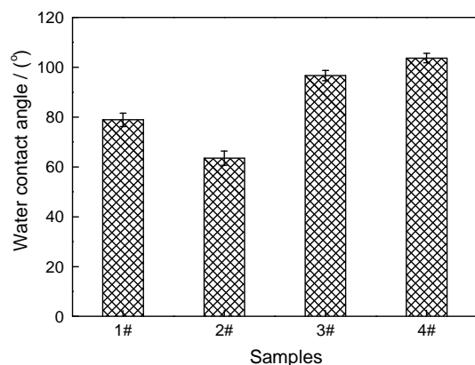
图1 样品接触角的变化
