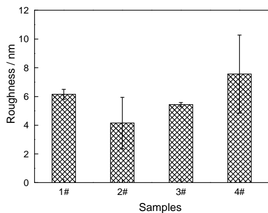
图5 不同样品的表面粗糙度变化 Fig.5 Roughness of difference samples
