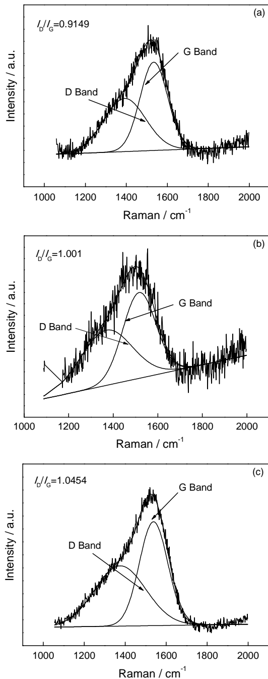
图3 PET沉积碳膜后的拉曼光谱图
